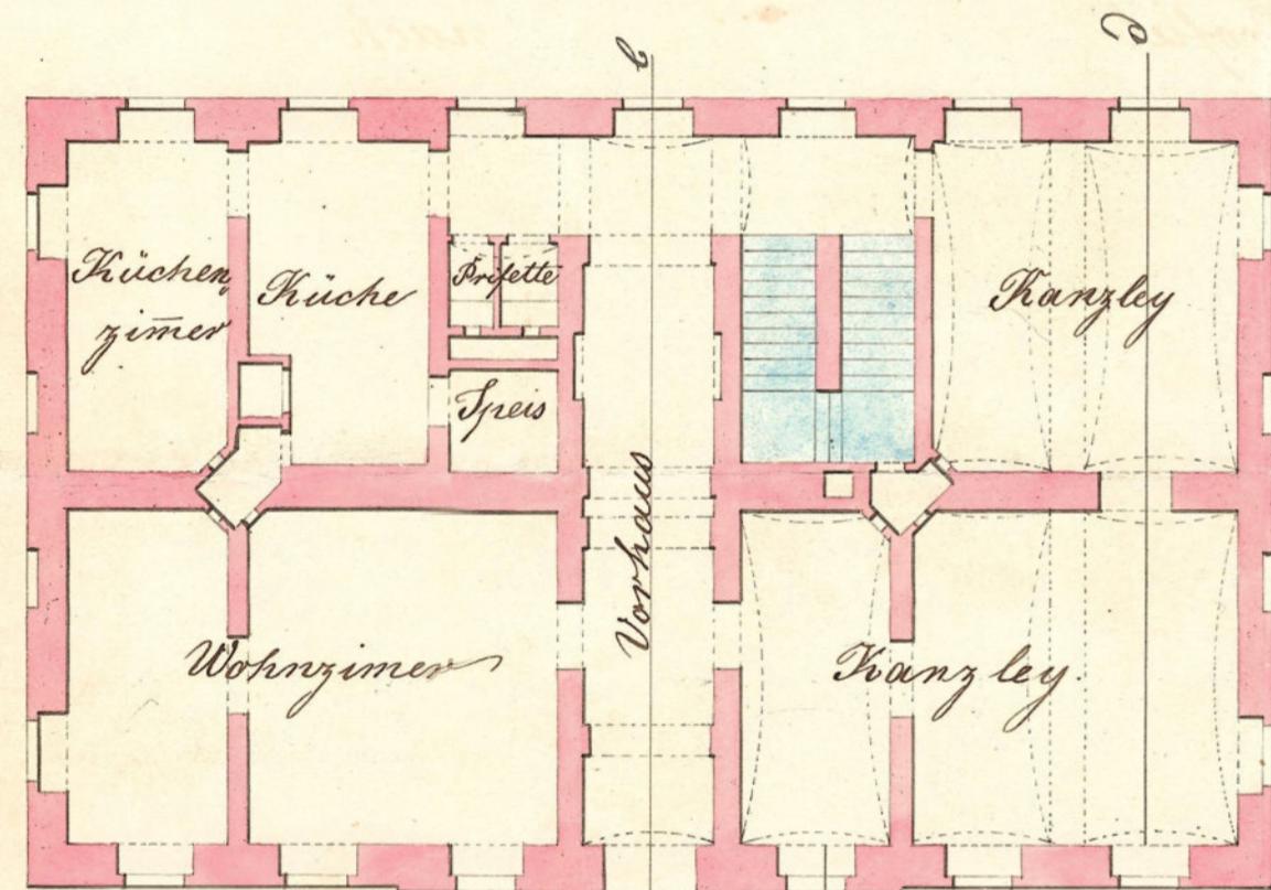
Grundriß zu ebener Erde
