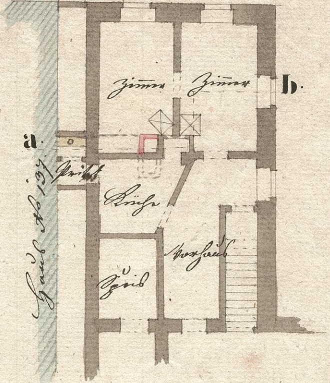
Grundriss des 2 ten Stockes
