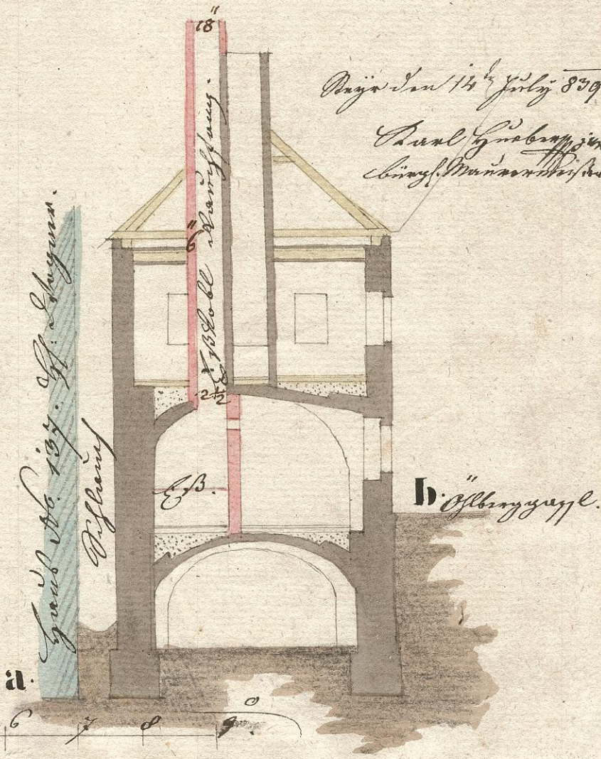
Profil durch a. b.
