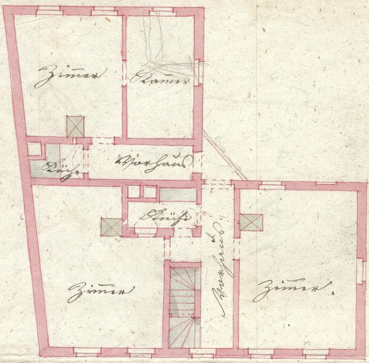
Grundriss des II ten Stockes
