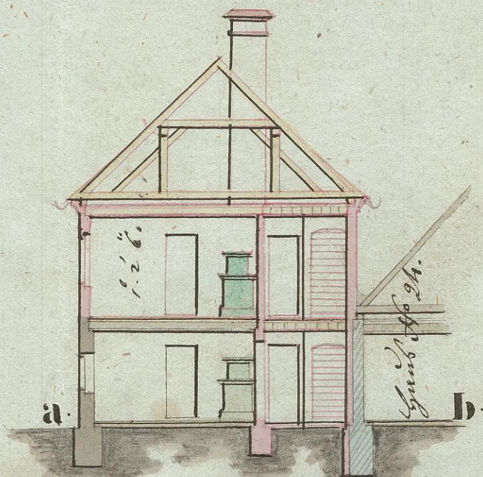
Profil durch a-b.
