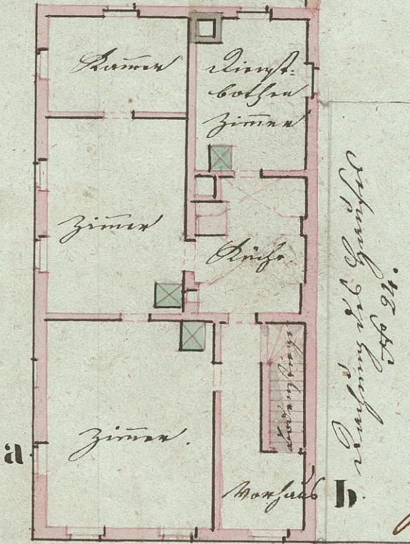
Grundriß des 1ten Stockes H. G. G. G. G.
