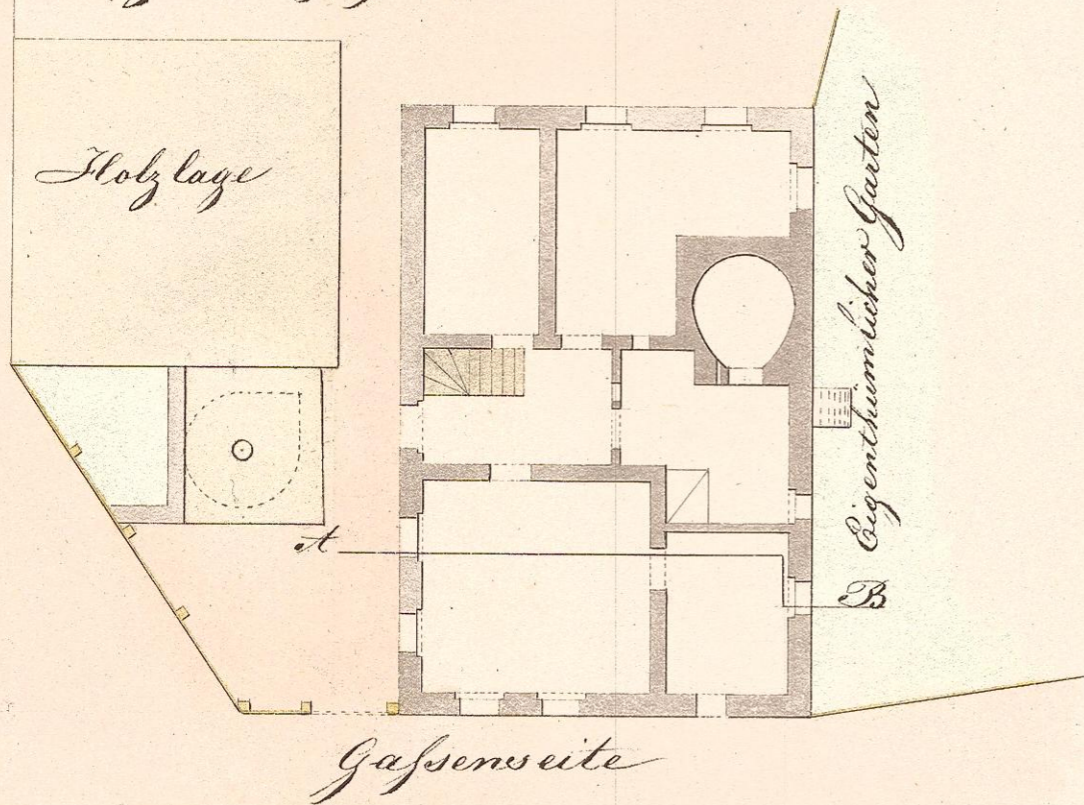
Grundriß zu ebner Erde
