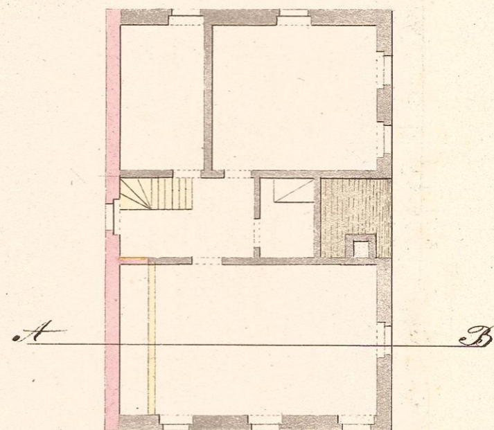
Grundriß des 1 ten Stockes
