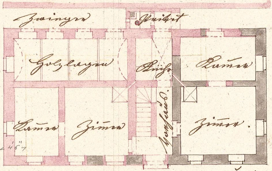
Grundriß zu ebner Erde
