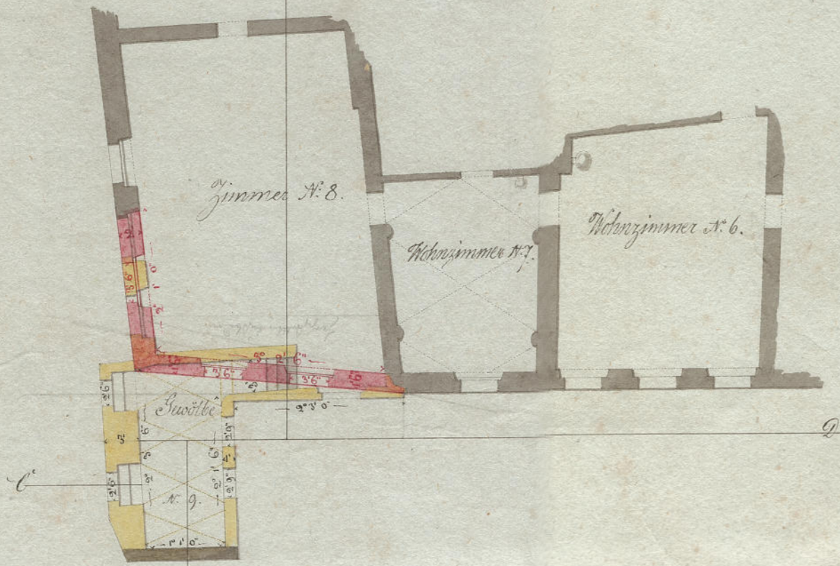
Grundriß des 1 ten Stockes.
