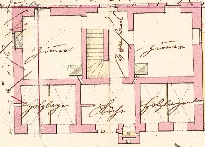
Grundriß zu ebener Erde.
