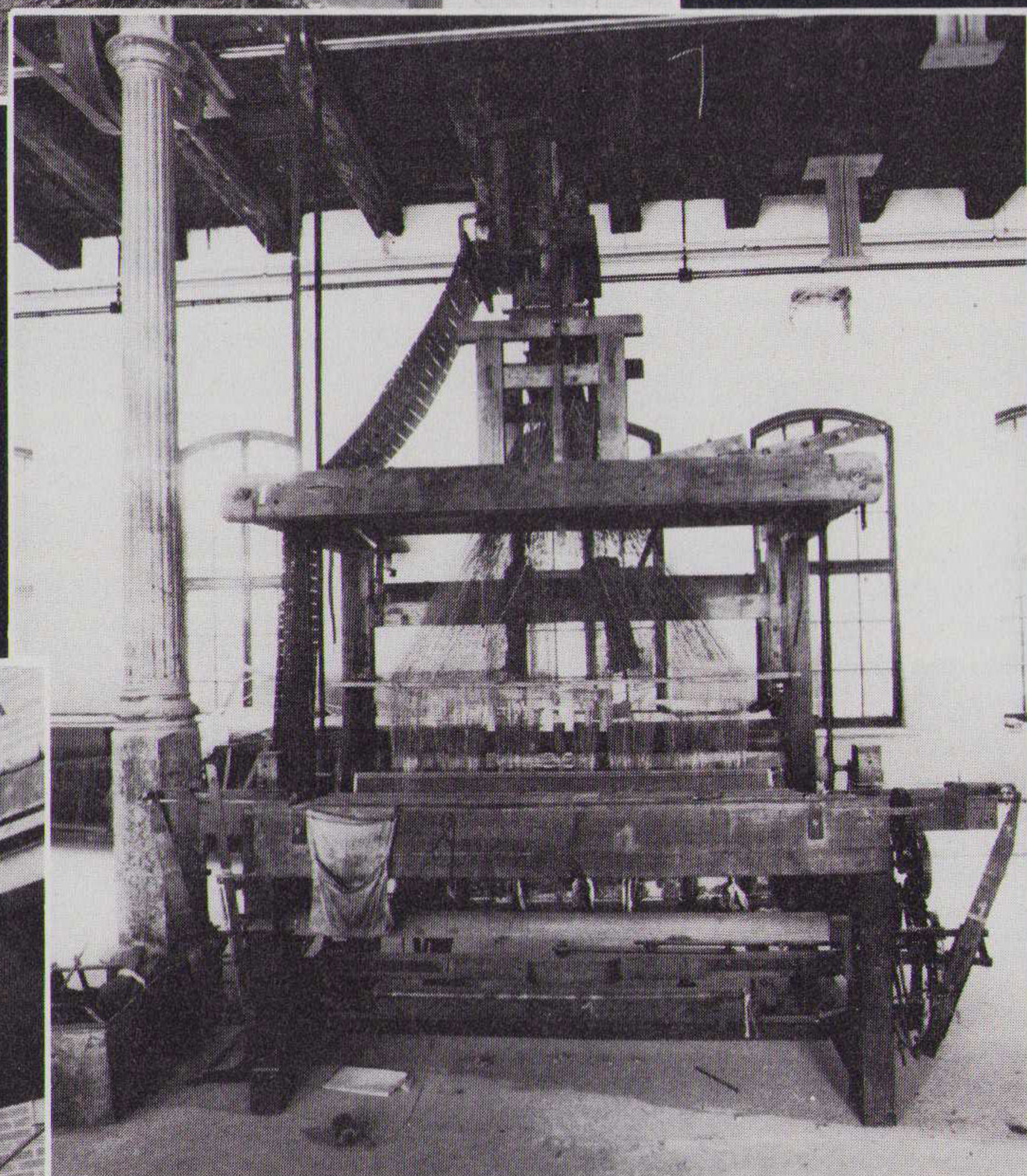
Dieser Jacquard-Webstuhl dient seit Ende des 18. Jahrhunderts für die Herstellung großflächig gewebter Musterungen.
