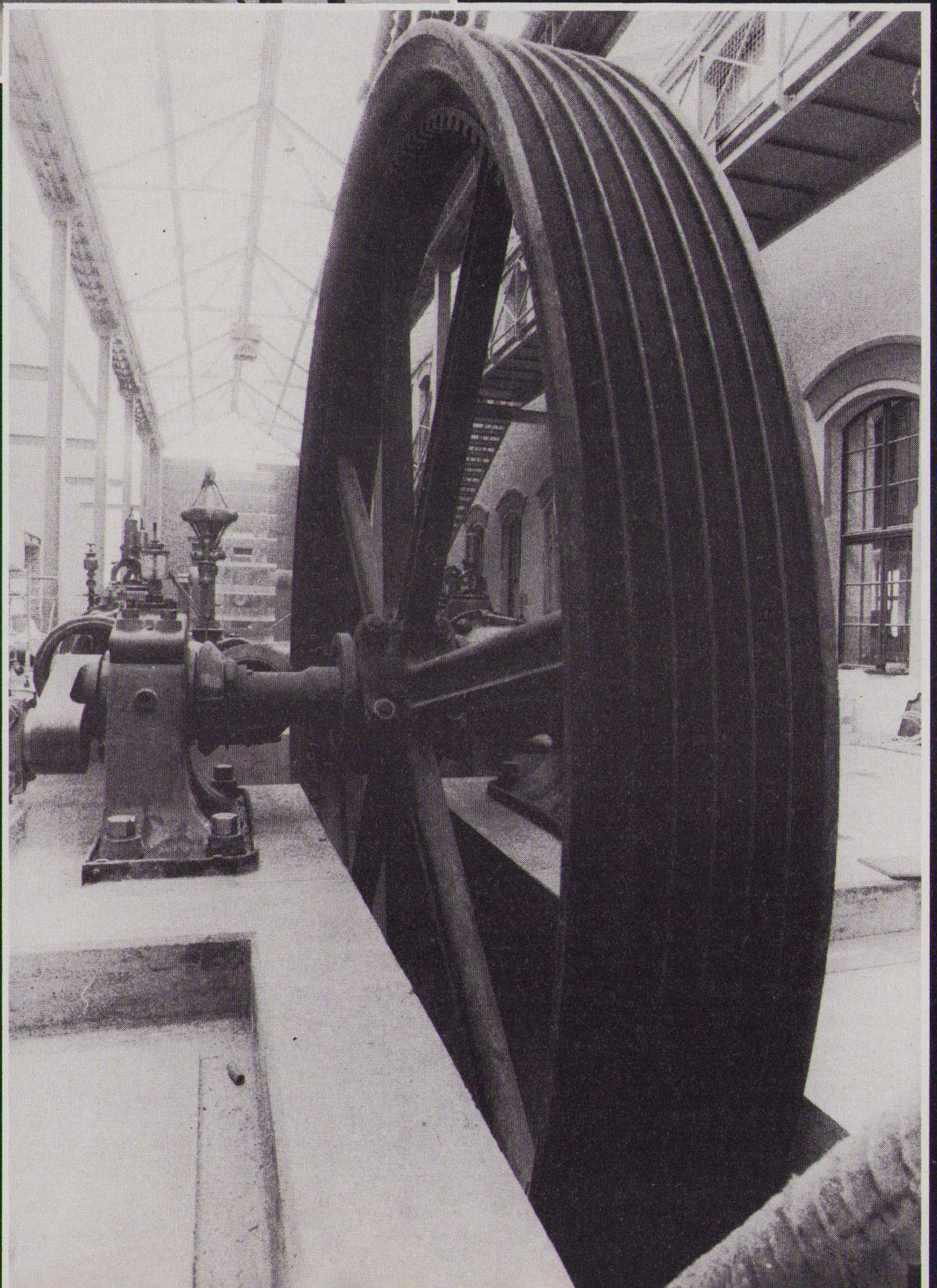
Das 4,5 Tonnen schwere Schwungrad der Dampfmaschine gibt die Antriebskraft über mächtige Seile an die Transmissionswelle weiter.
