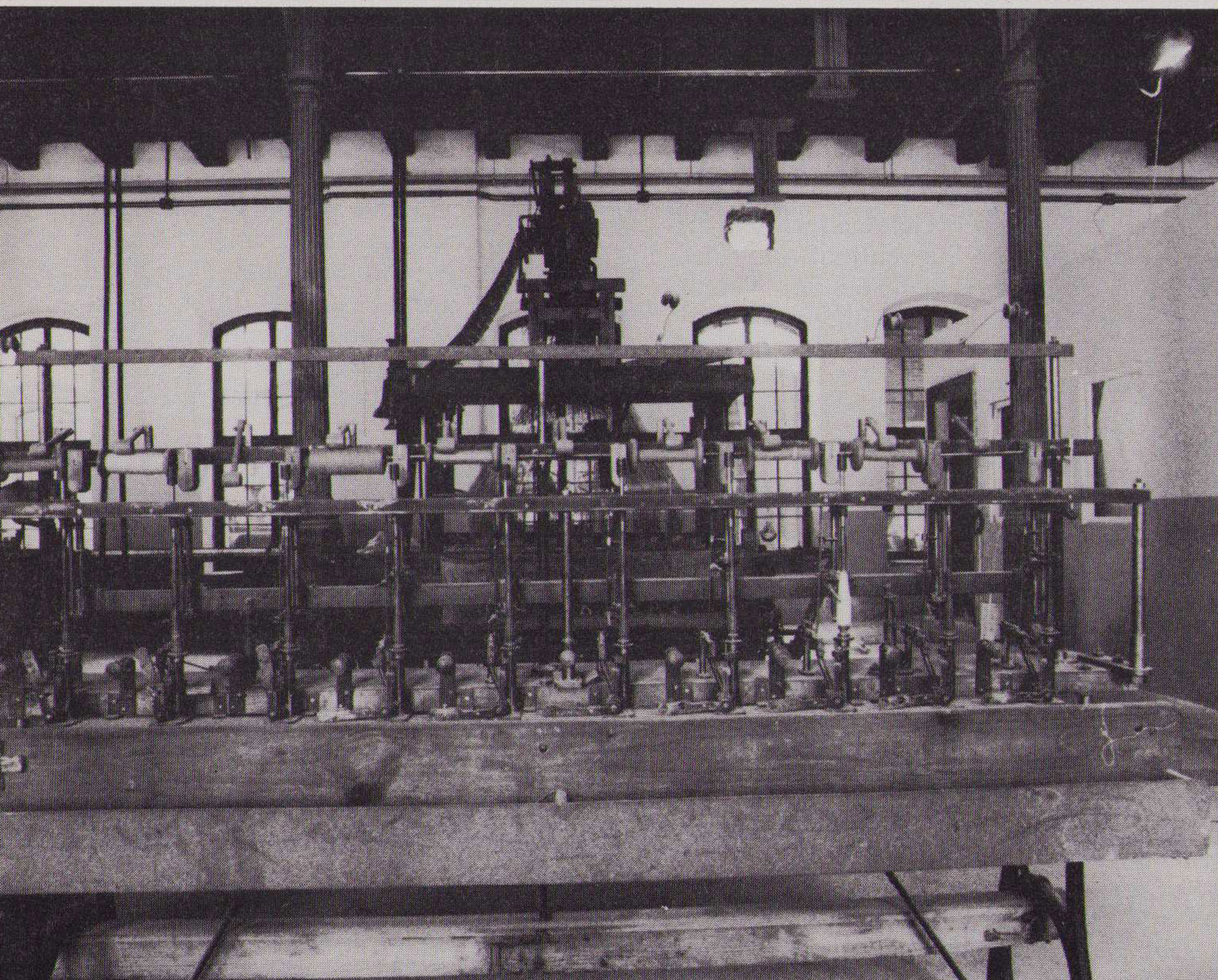
Eine Schuß-Spulenmaschine – Vorwerk zum Weben.
