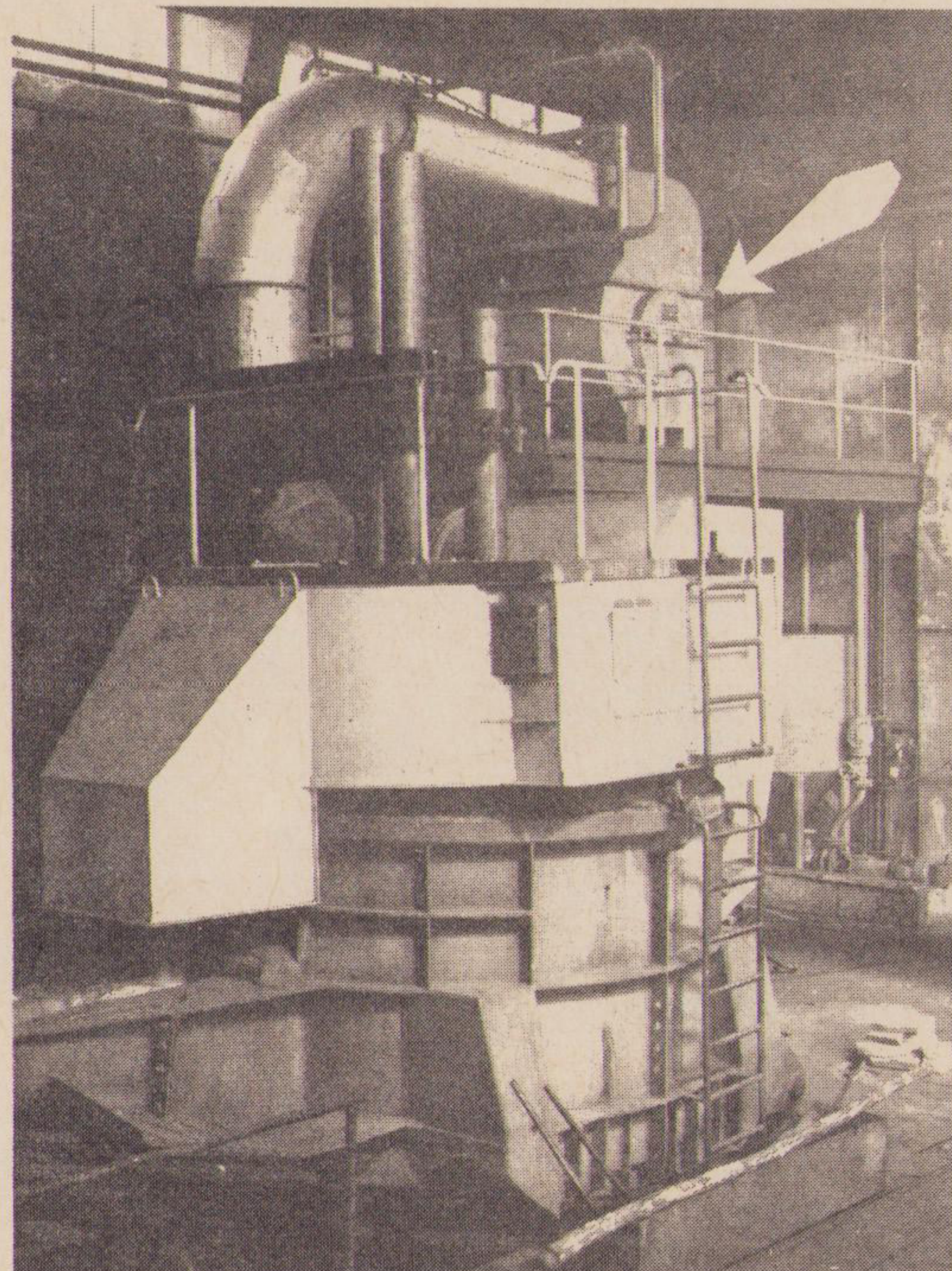
NASSABSCHNEIDER (ENTSTAUBUNGSANLAGE) EINES LICHTBOGENOFENS (Pfeil) GUSSWERK II
